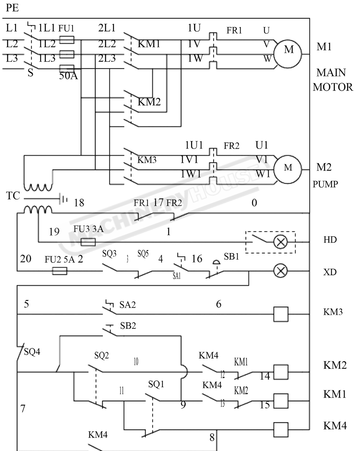
WIRINGDIAGRAM
